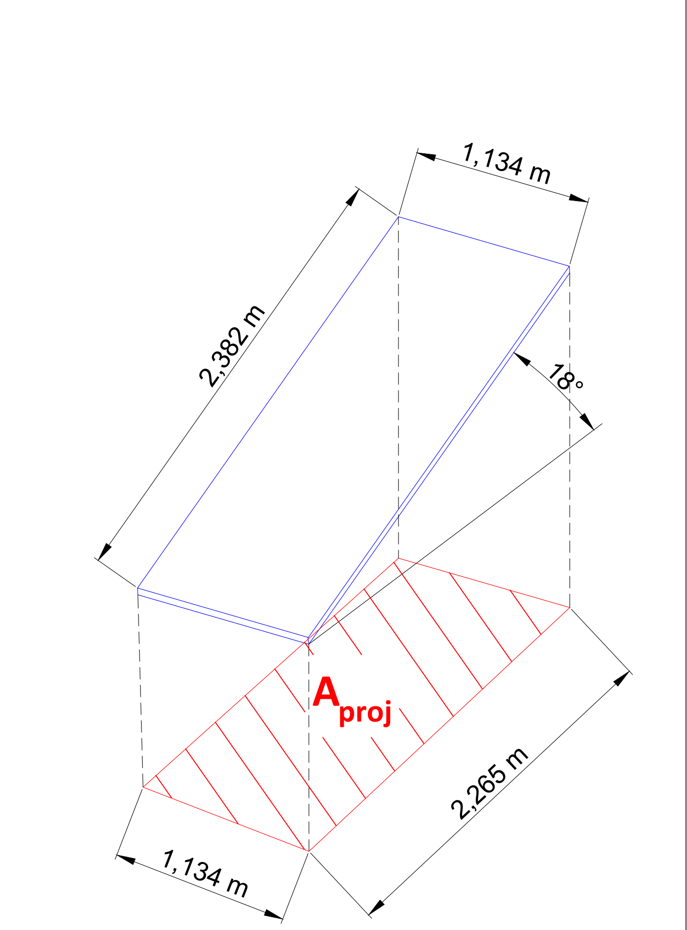
PV-Modul (Grundfläche)
